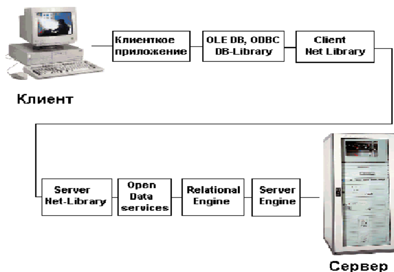
Сурет 2.3 – Клиент-сервер архитектурасы
