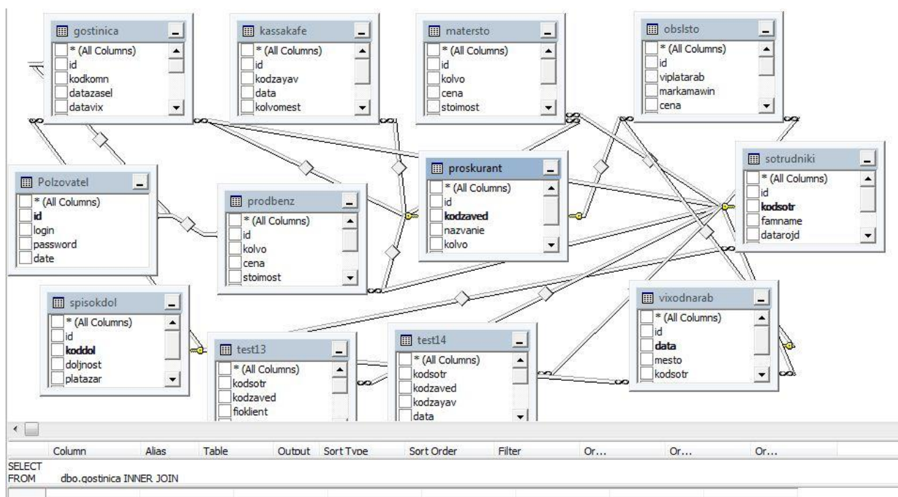
Сурет 3.1 – ДҚ диаграммасы
