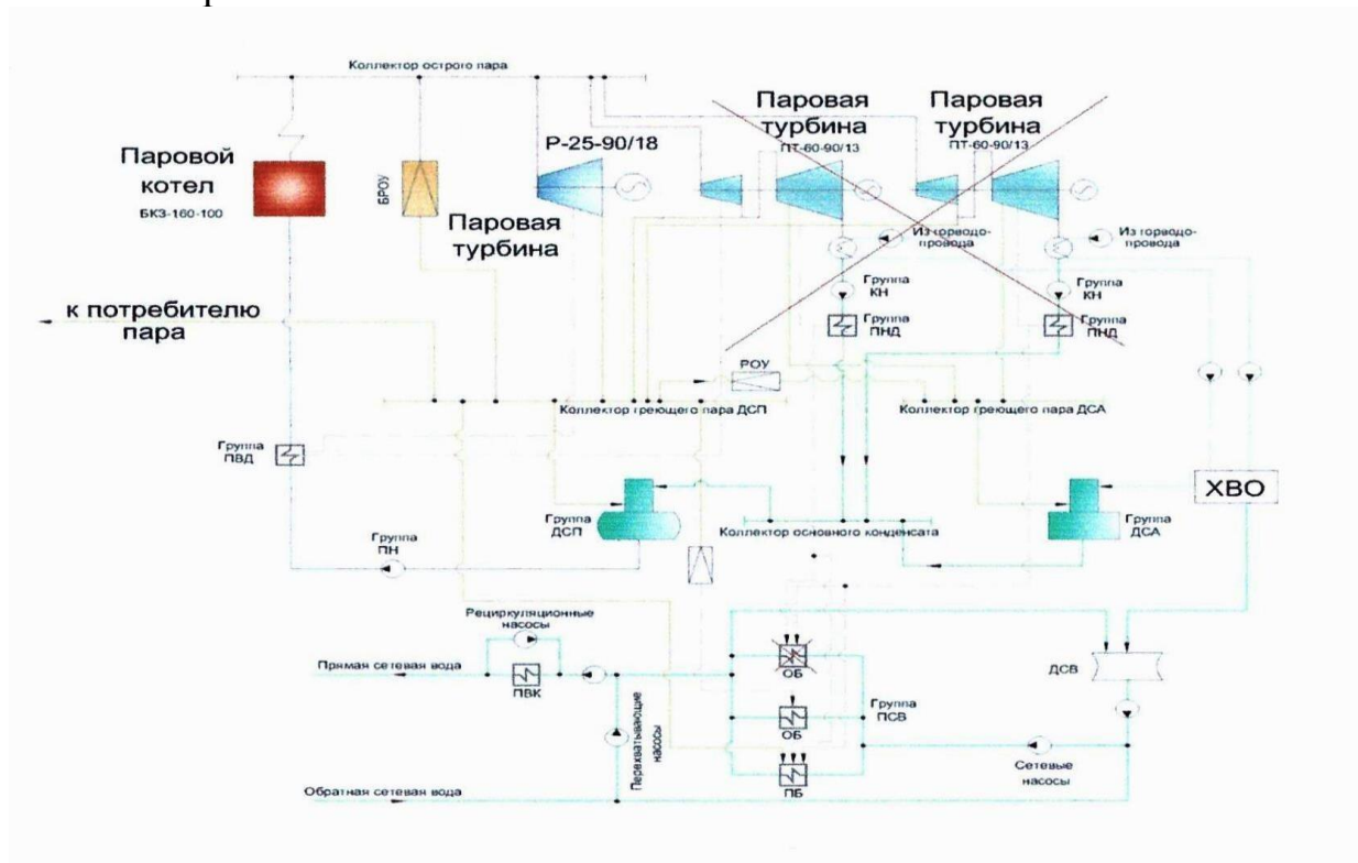
Рисунок 2.1 – Тепловая схема АО АлЭС ТЭЦ-1
