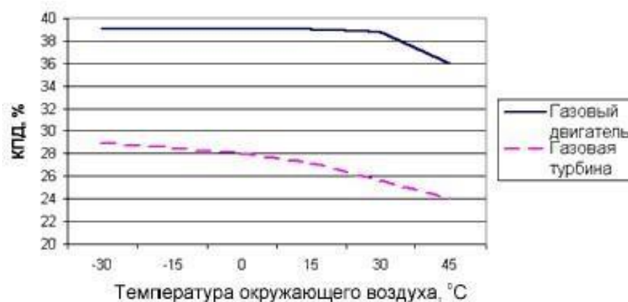
Рисунок 2.3 - График зависимости электрического КПД газовой турбины от температуры окружающего воздуха
