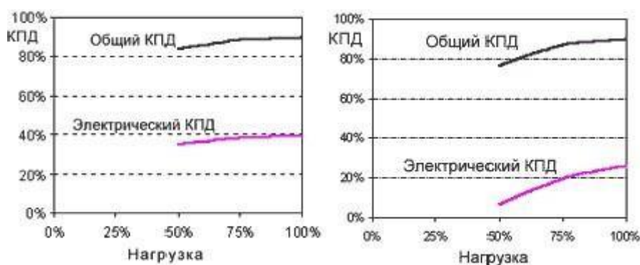
Рисунок 2.2 - Графики зависимости КПД от нагрузки
