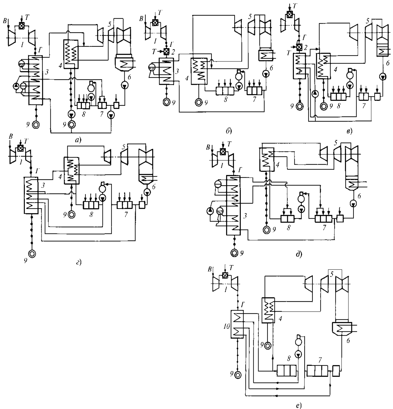
а — подвод пара в холодную линию системы промперегрева; б - подвод пара в горячую линию системы промперегрева; в — подвод пара в линию свежего пара; г — подвод пара в промежуточную точку парового тракта котла; д — вытеснение пара из узла регенерации паровой турбины паром из котла-утилизатора; е — установка газовойодяных подогревателей (ГВП) конденсата и питательной воды взамен узла регенерации паровой турбины; 1 — газовая турбина; 2 — горелки котла-утилизатора; 3 — котел-утилизатор; 4 — котел надстраиваемого блока; 5 — паровая турбина; 6 — конденсатор; 7, 8 — подогреватели соответственно низкого и высокого давления; 9 — дымовая труба; 10 -ГВП низкого и высокого давления; Т — топливо; В — воздух; Г — газы
