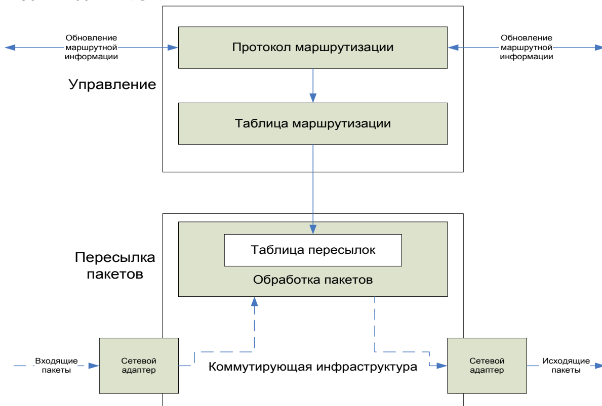
Рисунок 2.3. Функциональные компоненты маршрутизации
