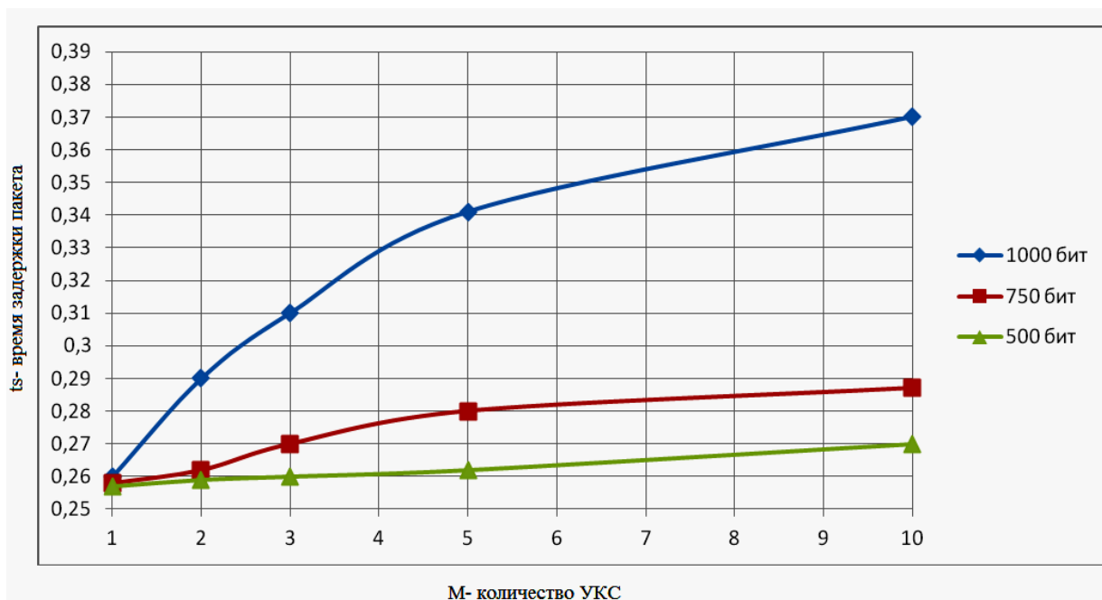
Рисунок 6.4 – Зависимость времени задержки пакета от количества УКС при разной длине пакета (Ts – время задержки пакета, сек.; M – количество УКС пропускной способности канала 128 Кбит/с)
