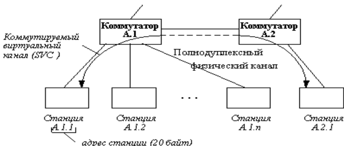
Рисунок. 2.1. Структурная схема сети NGN с ATM
