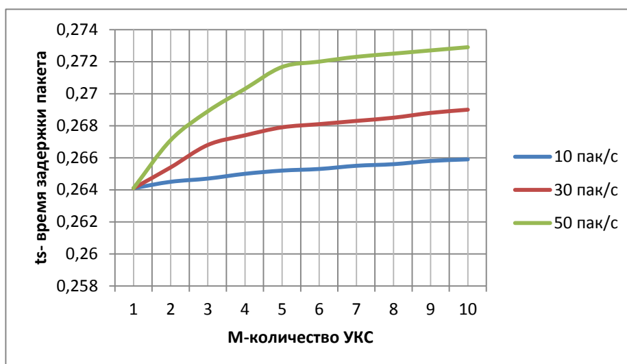
Рисунок 6.2 – Зависимость времени задержки пакета от количества УКС при разной интенсивности генерирования пакетов ( T_s – время задержки пакета, секунды; M – количество УКС пропускной способности канала 128 Кбит/с и длине пакета 1000 бит)
