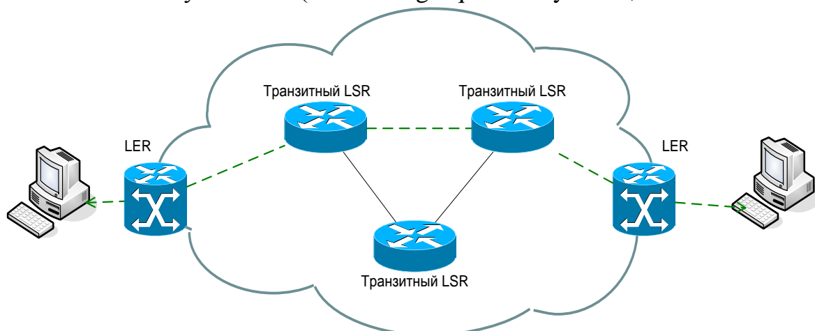
Рисунок 2.2 – Архитектура сети MPLS
