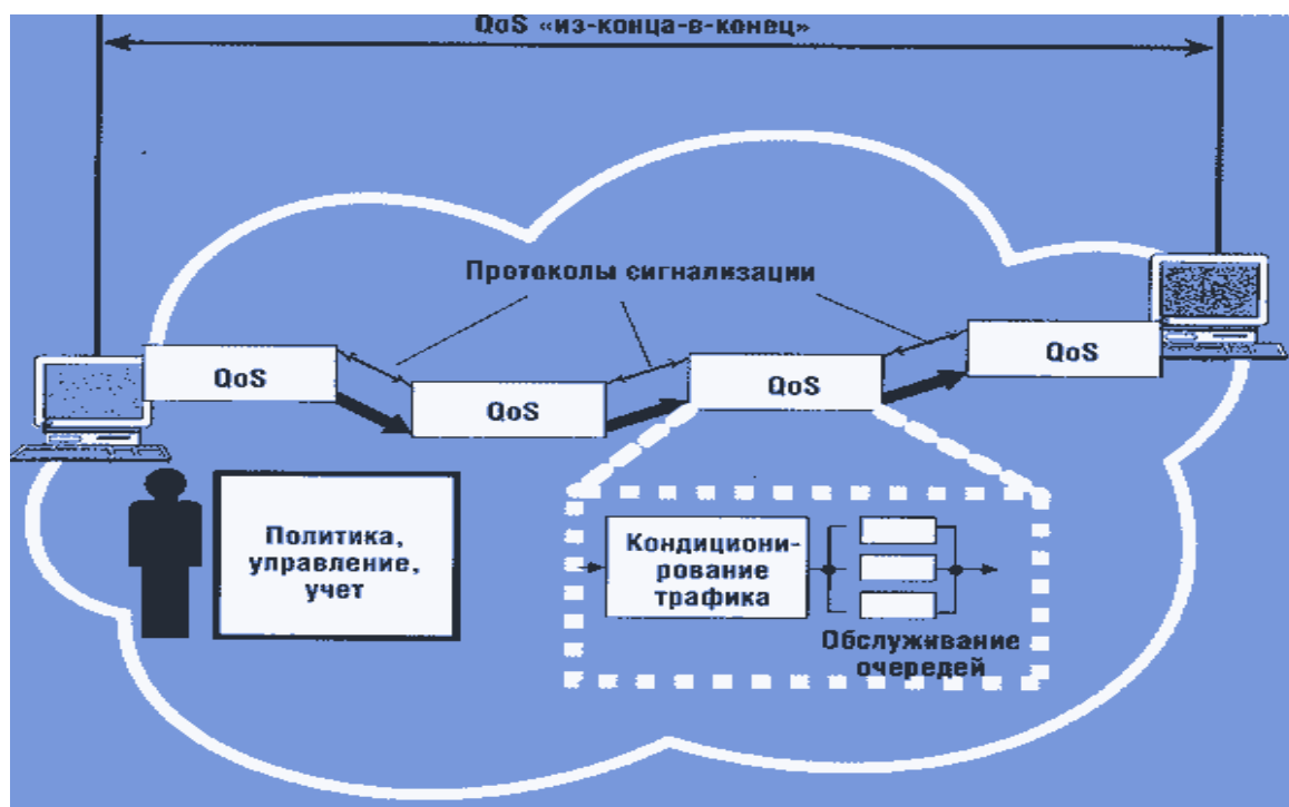
Рисунок 3.2 – Типовая архитектура службы QoS с элементами трех основных видов:
