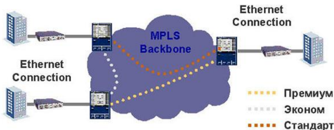
Рисунок 3.1 – Виды трафика согласно класса обслуживания в сетях NGN
