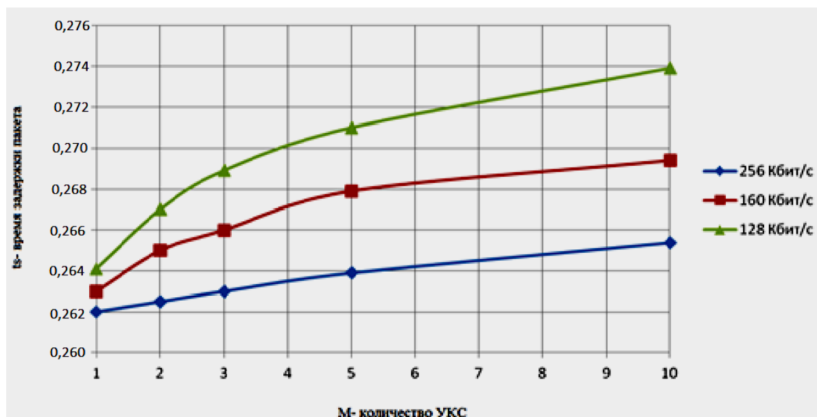
Рисунок 6.3 – Зависимость времени задержки пакета от количества УКС при разной пропускной способности канала ( T_s – время задержки пакета, сек.; M – количество УКС при интенсивности генерирования пакетов равной 50 пак./с и длине пакета 1000 бит)
