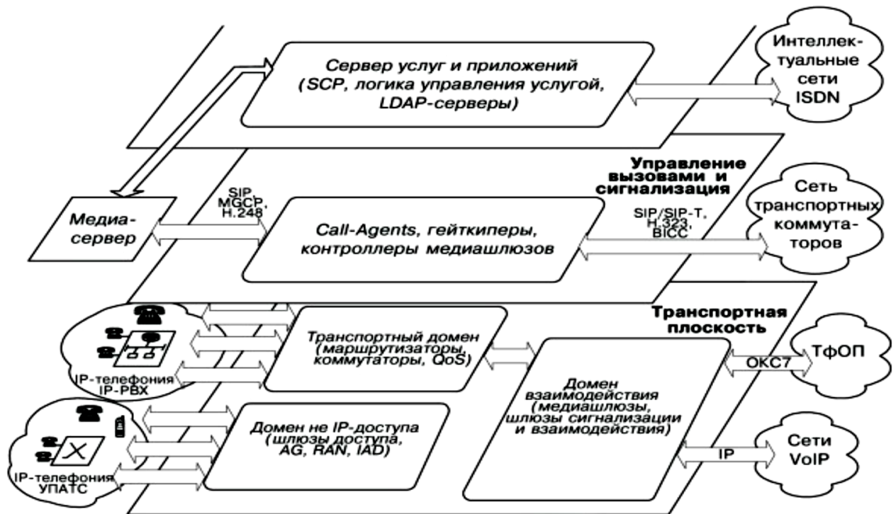
Рисунок 2. Структура SoftSwitch
