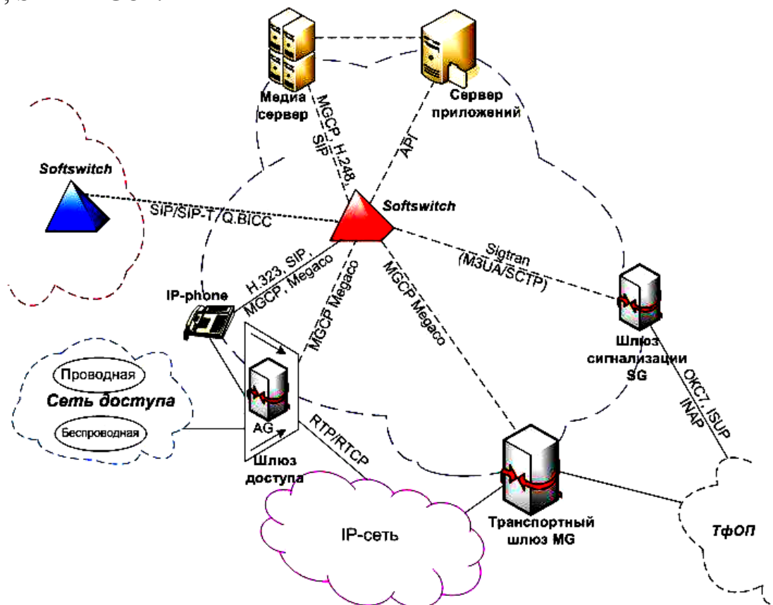
Рисунок 1.1 – Схема организации сети NGN
