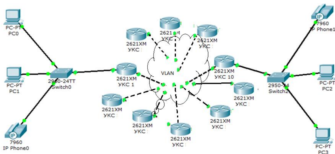
Рисунок 6.5 – Модель исследуемой телекоммуникационной сети с 10 УКС
