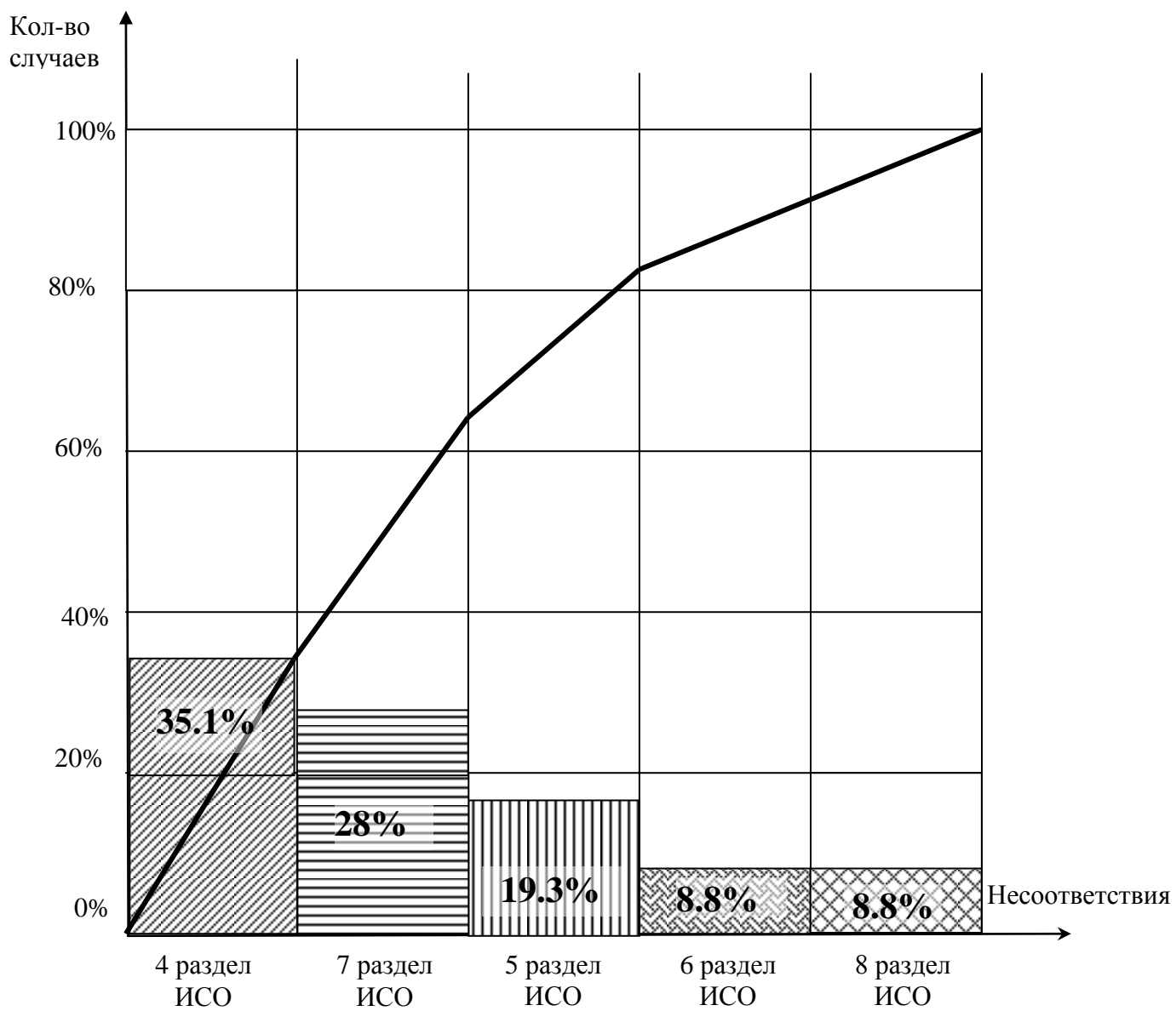
Диаграмма Парето
